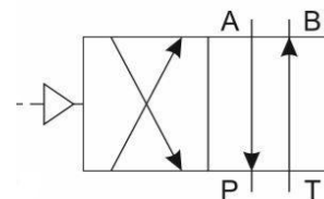
Valvola direzionale idraulica 4/2 Cetop03 ad azionamento pneumatico Hydraulic directional valve 4/2 Cetop03 pneumatically operated
